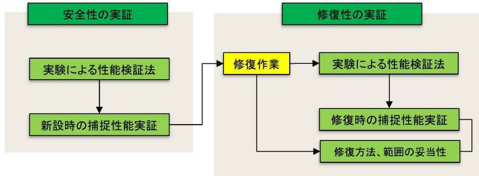
強靱防護網 安全性・修復性 実証フロー
